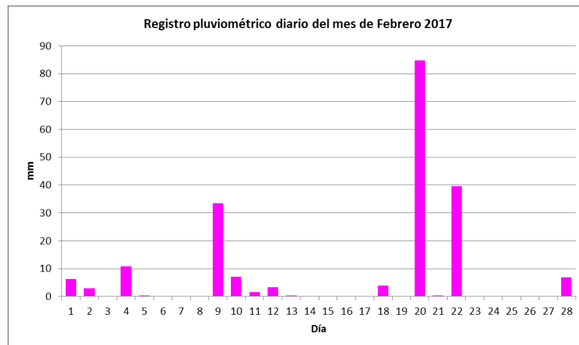
Gráfico N° 1: Precipitaciones diarias de Febrero de 2017.
