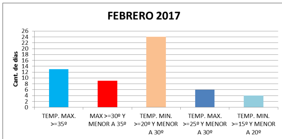
Gráfico N° 4: Detalle de cantidad de días con temperaturas máximas superiores a 35°, entre 30° y 35° y entre 25° y 30°C; y temperaturas mínimas entre 15° y 20° y entre 20° y 30°C de Febrero de 2017.
