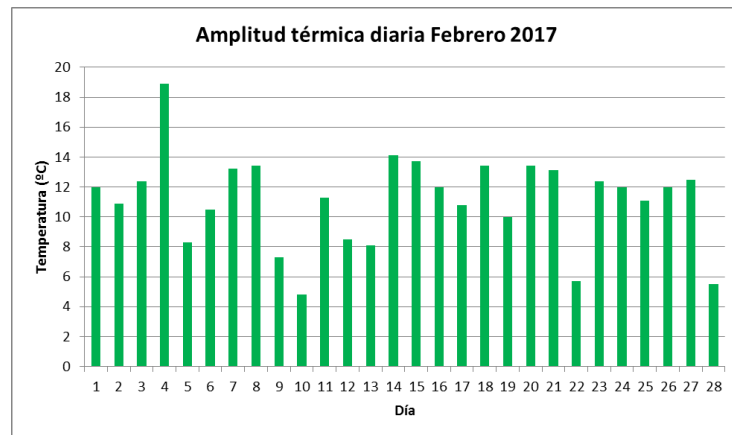
Gráfico N° 5: Amplitud Térmica diaria de Febrero de 2017.
