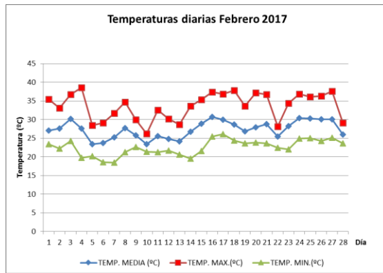
Gráfico N° 2: Temperaturas diarias.
