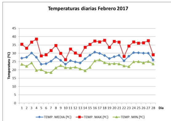
Gráfico N° 2: Temperaturas diarias.
