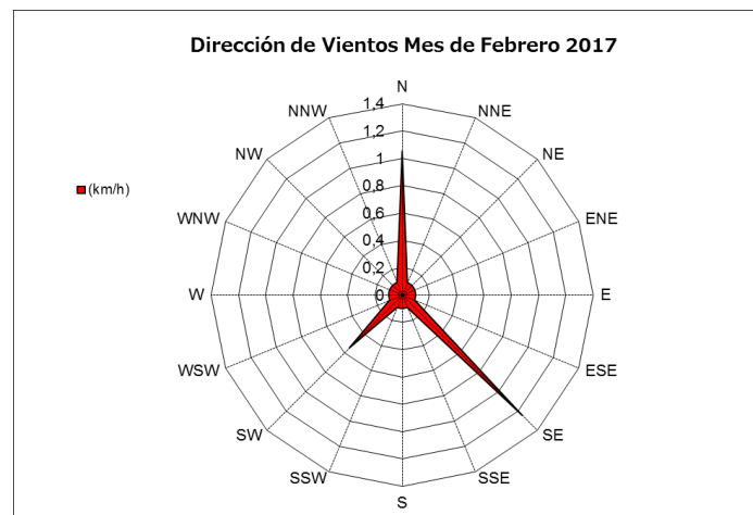
Gráfico N° 6: Rosa de vientos correspondientes al mes de Febrero de 2017.
